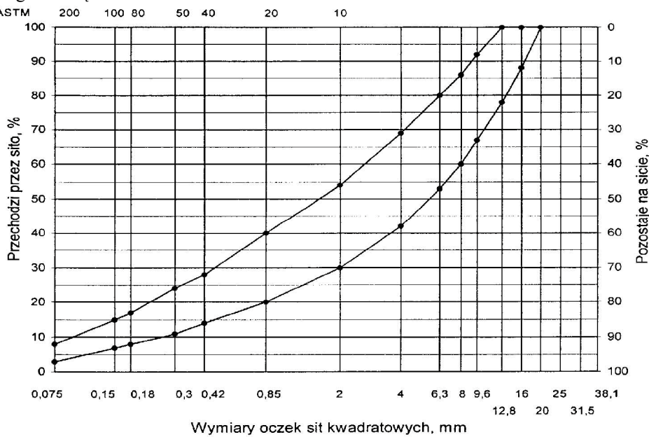
Rys. 5. Krzywe graniczne uziarnienia mieszanki mineralnej BA od 0 do 16 mm do warstwy wiążącej nawierzchni drogi o obciążeniu ruchem KR1-2
