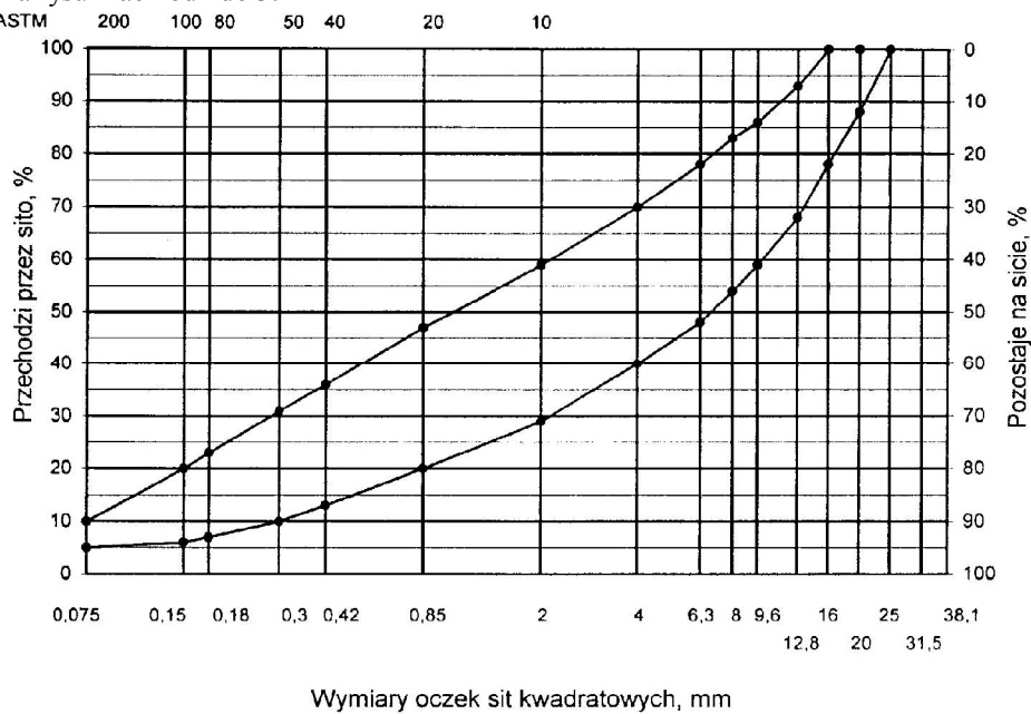
Rys. 1. Krzywe graniczne uziarnienia mieszanki mineralnej BA od 0 do 20 mm do warstwy ścieralnej nawierzchni drogi o obciążeniu ruchem dla KR 1-2
