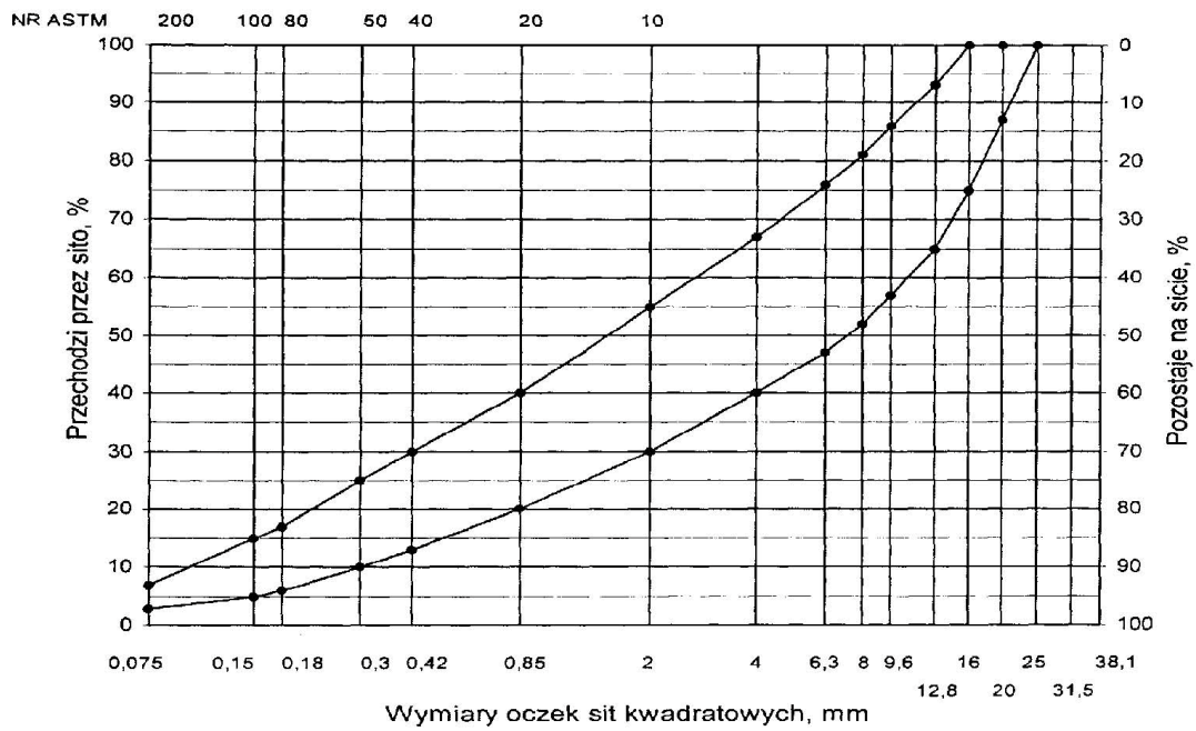
Rys. 4. Krzywe graniczne uziarnienia mieszanki mineralnej BA od 0 do 20 mm do warstwy wiążącej nawierzchni drogi o obciążeniu ruchem KR1-2
